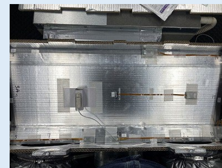
SAチャンバー内センサー貼付状況
